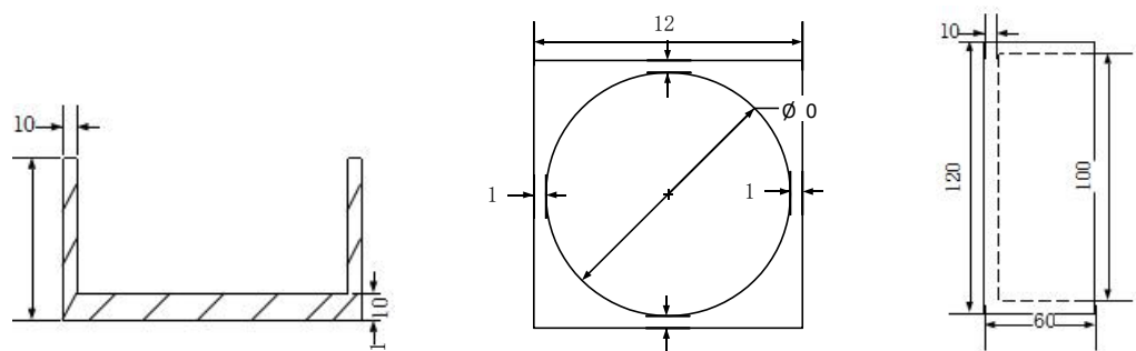
图 8 矿物桶模型尺寸
