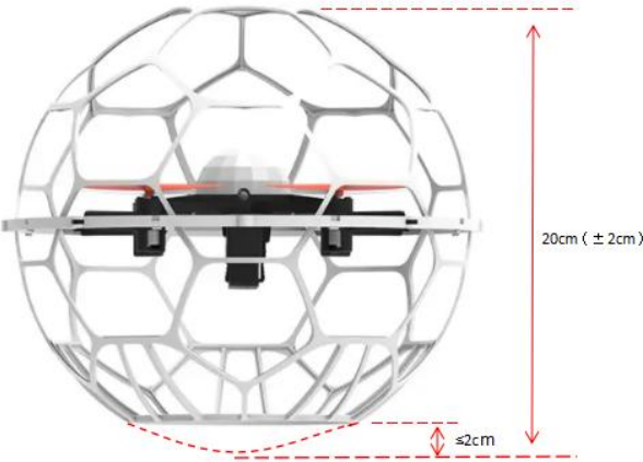
图 4 无人机球外框架示意图
