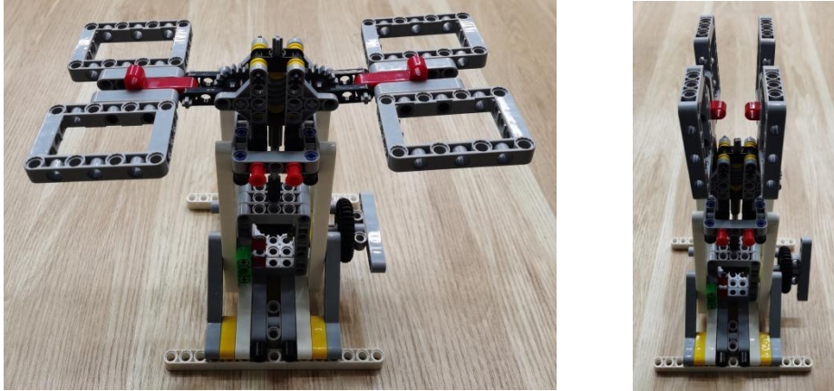
图2 车身塑型的初始状态及完成状态
