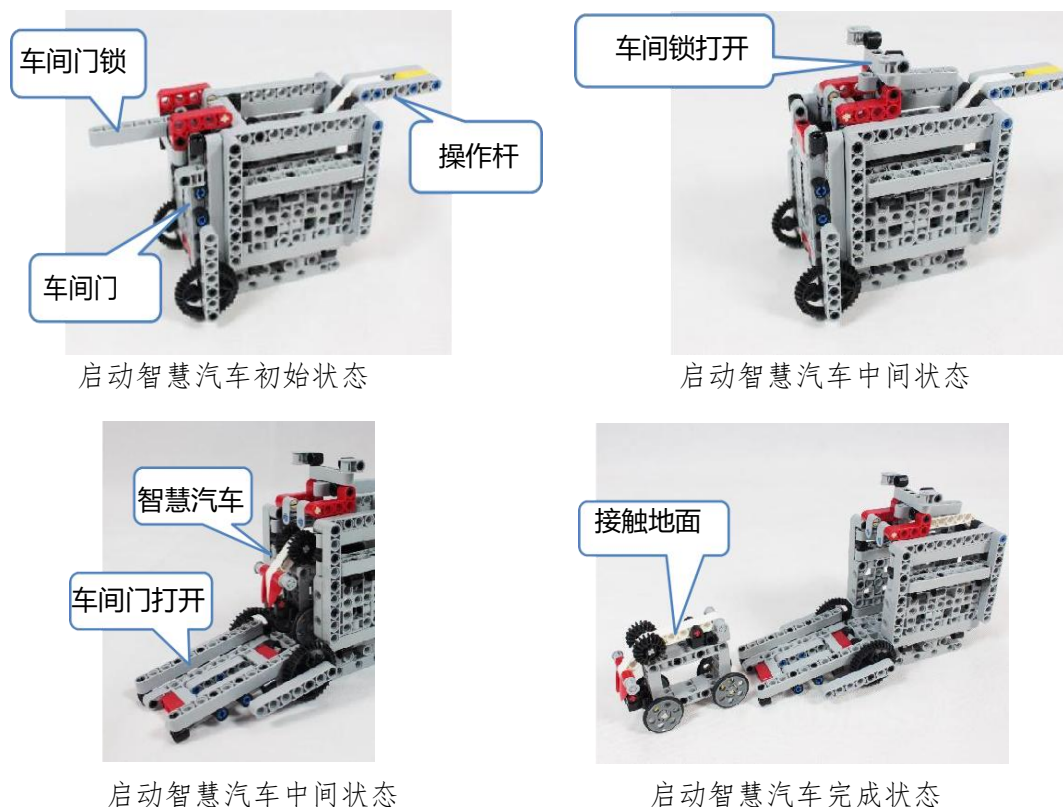
图6 总装出厂的初始状态及完成状态
